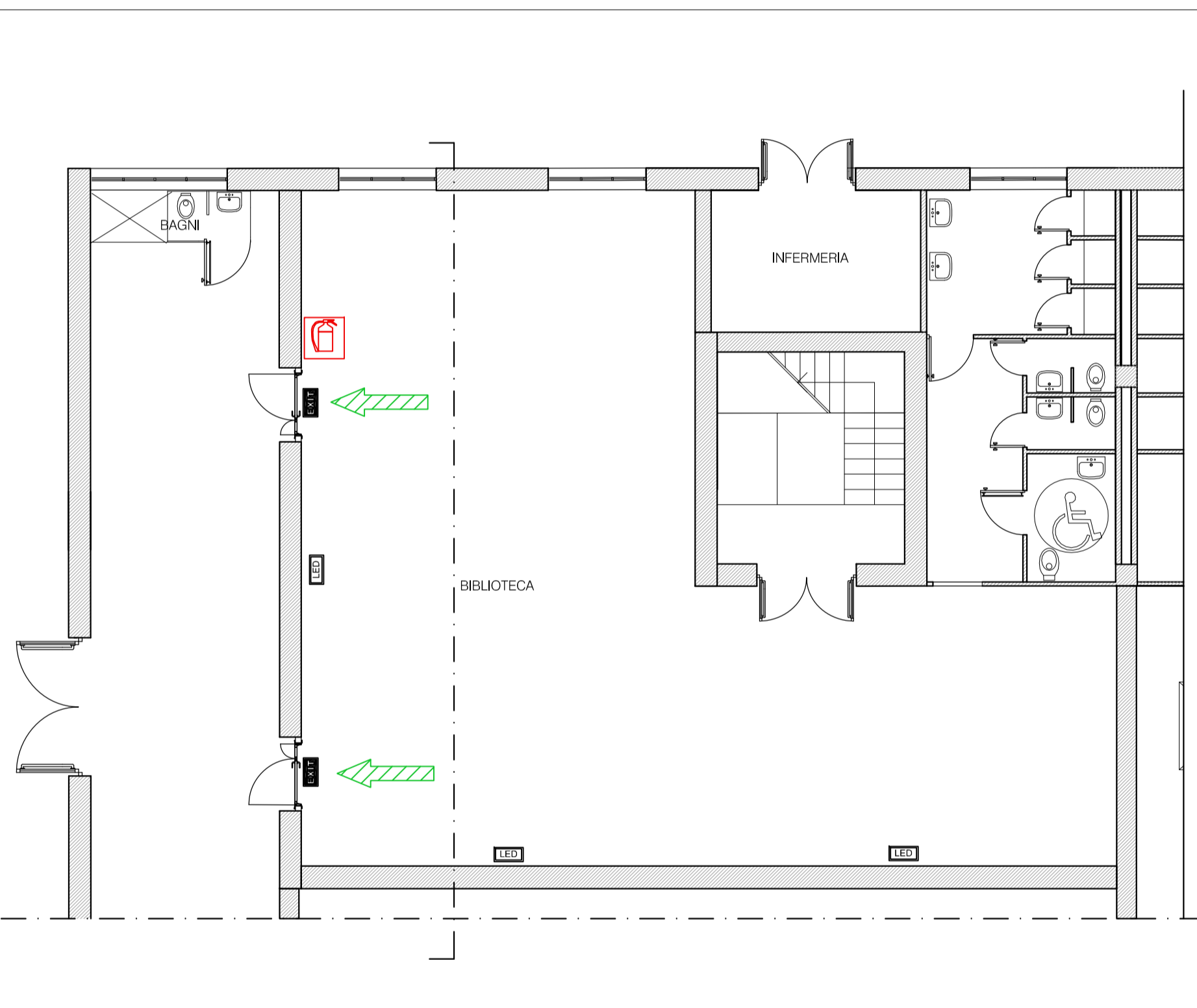
PROGETTO: PIANTE LIVELLO CORTILE Scala 1:100
