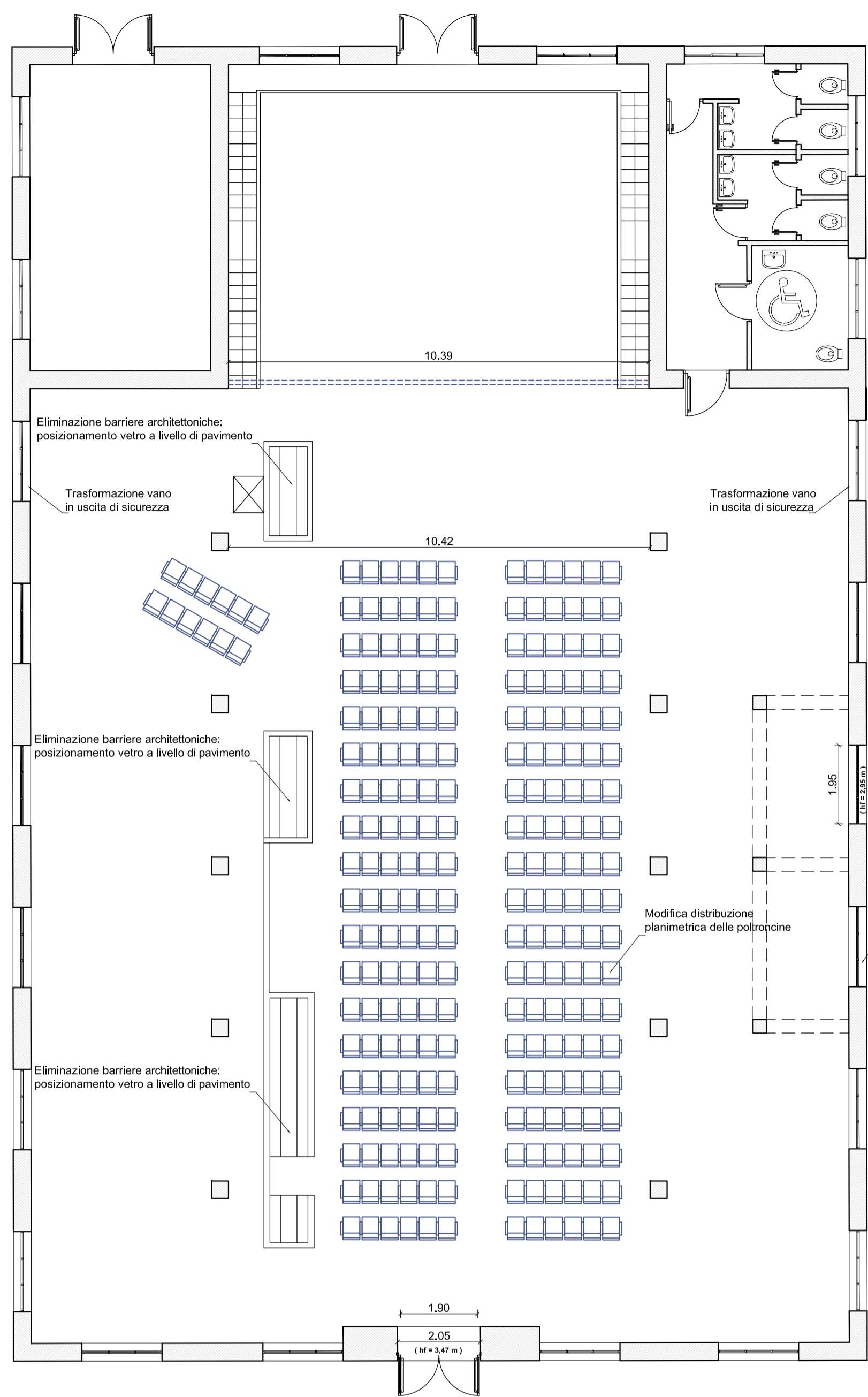
RILIEVO: PIANTA AULA MAGNA CON INDICAZIONE INTERVENTI Scala 1:100
