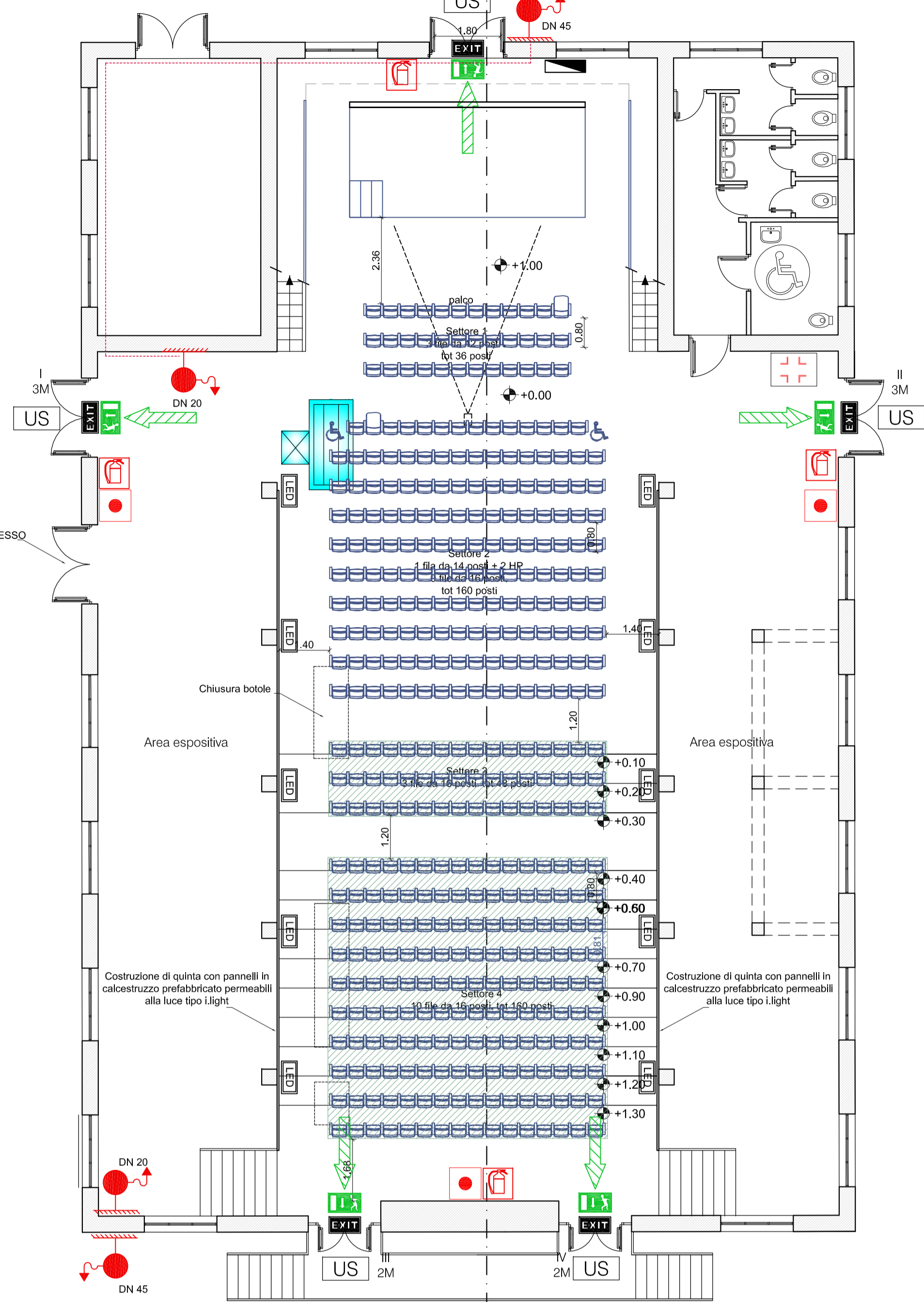
PROGETTO: PIANTA AULA MAGNA Scala 1:100
