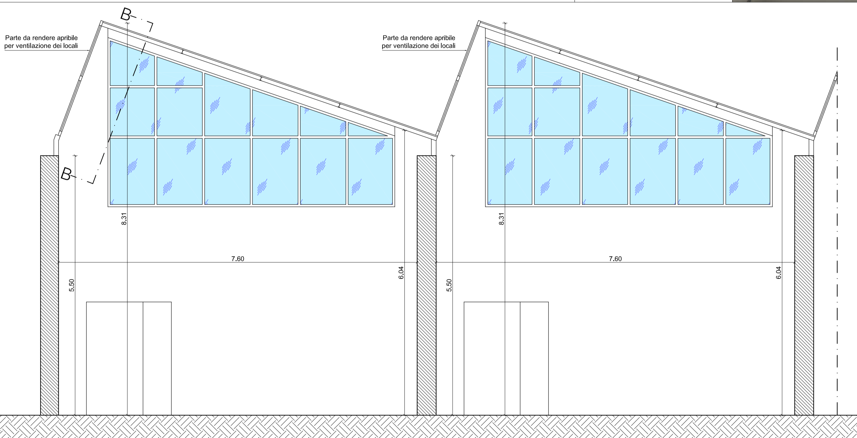
SEZIONE TRASVERSALE A-A - Scala 1:50
