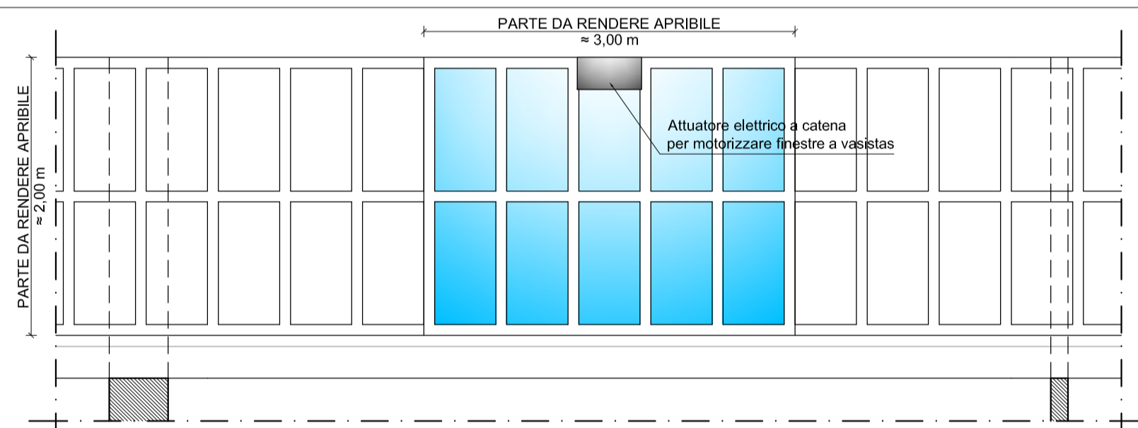
DETTAGLIO DI VENTILAZIONE - SEZIONE B-B - Scala 1:50
