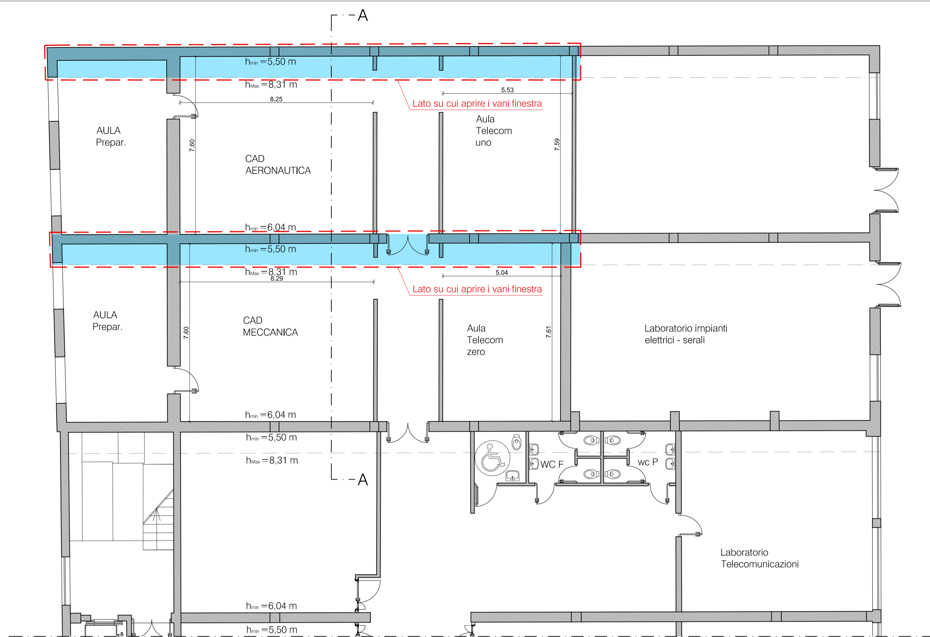
PIANTA PIANO TERRA: RILIEVO CON INDICAZIONE DEGLI INTERVENTI Scala 1:100
